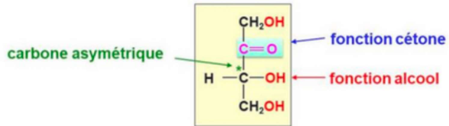
D-érythrulose
